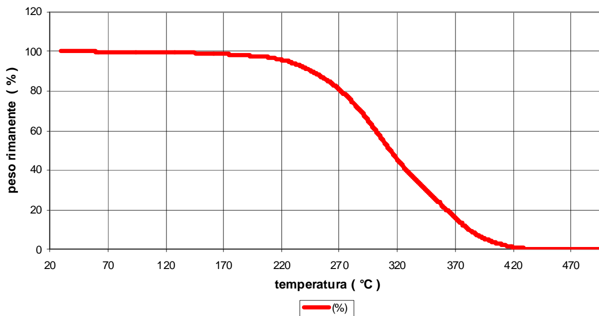
perdita di peso% Resinol RTC polimerizzato sotto stress dinamico (5°C/min)
